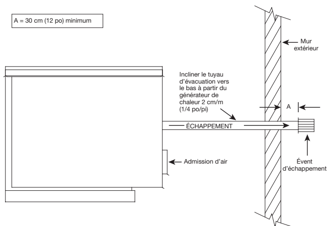
Évacuation intérieure standard - horizontale
