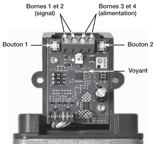
Vanne de gaz modulante EXA (couvercle retiré)
