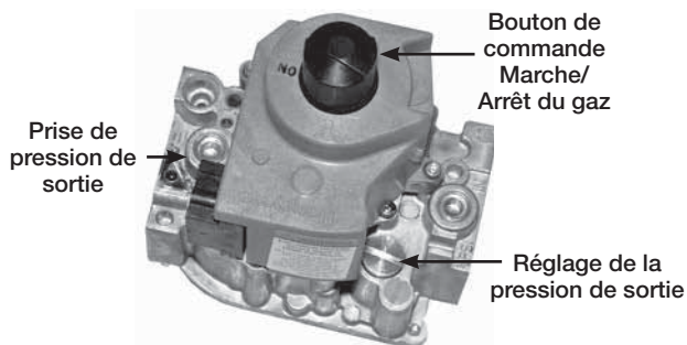
Vanne de gaz mono-niveau typique
