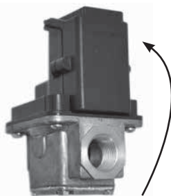
L'ajustement des allures de chauffe basse et haute se fait sur le circuit imprimé derrière le capot amovible
