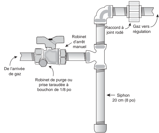
Raccordement de tuyauterie d'arrivée de gaz typique
