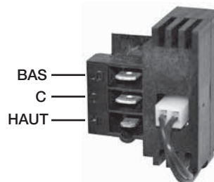
Détail du bornier
