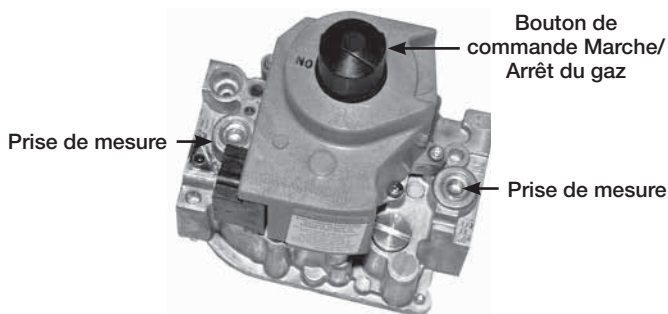
Vanne de gaz mono-niveau typique
